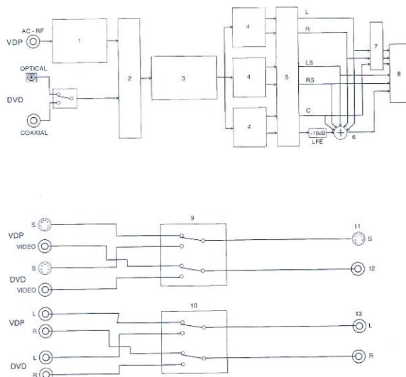
Blokschema ED-901
